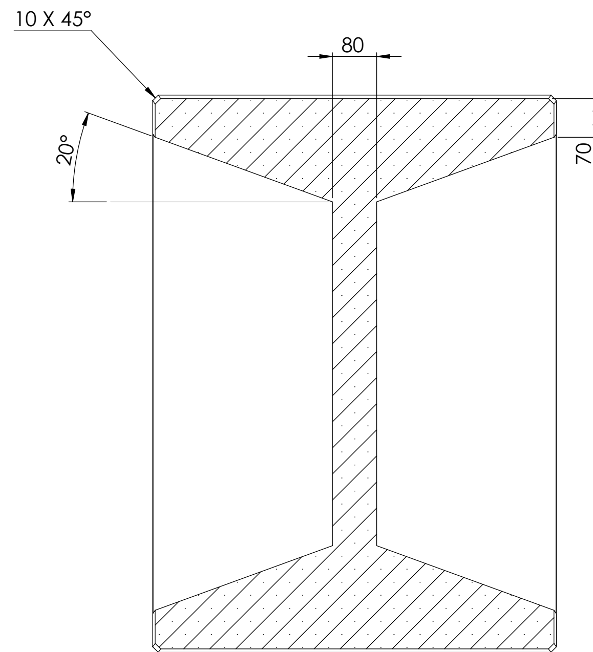
SEÇÃO A-A ESCALA 1 : 7
